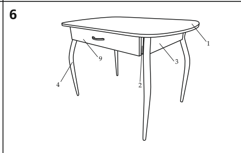
Собрать царговый пояс и скрепить вместе с каркасом для ящика.
